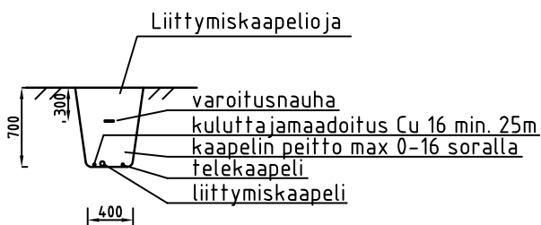
Kuva 1. Kaapeliojan poikkileikkaus
